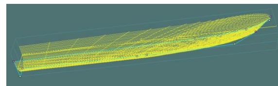
Gambar 2. Pemodelan Kapal Jukung dengan Software Maxsurf
