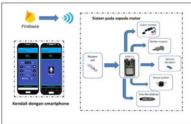
Gambar 2. Blok Diagram Rangkaian
