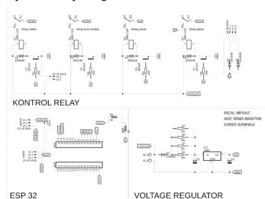
Gambar 3. Skematik Rangkaian
