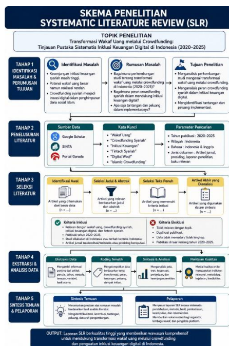
Gambar 1. Skema penelitian
