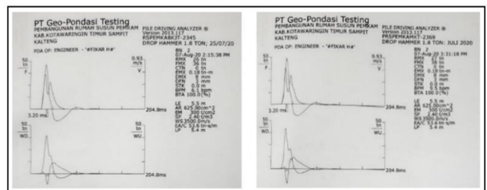
Gambar 3. Grafik hasil pengujian PDA test nomor tiang PRSPEMKAMKT-2345 dan tiang PRSPEMKAMKT-2369 Rusun Pemkab Kotim
