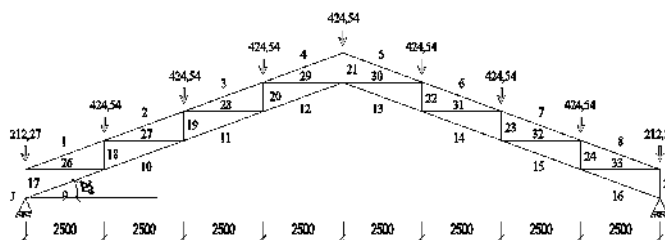
Gambar 6. Beban hidup (kg) pada rangka atap bentang 20 m
