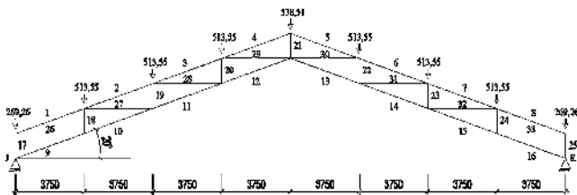
Gambar 8. Beban mati (kg) pada rangka atap bentang 30 m
