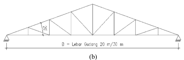
Gambar 1 Kuda-kuda rangka baja model paralel (a) dan model segitiga (b)
