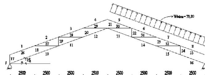
Gambar 7. Beban angin (kg) pada rangka atap bentang 20 m
