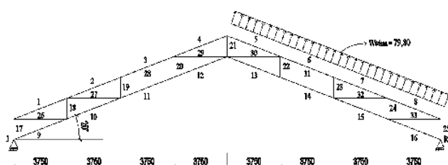
Gambar 10. Beban angin (kg) pada rangka atap bentang 30 m
